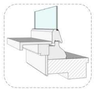
kozijn C1
