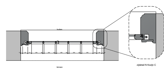
kozijn C
